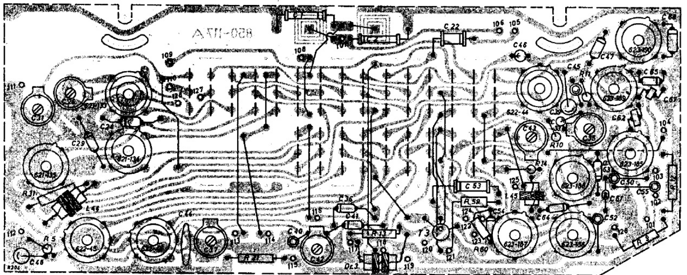
Obere Platte — Bestückungsseite Upper Plate — Component Side View
